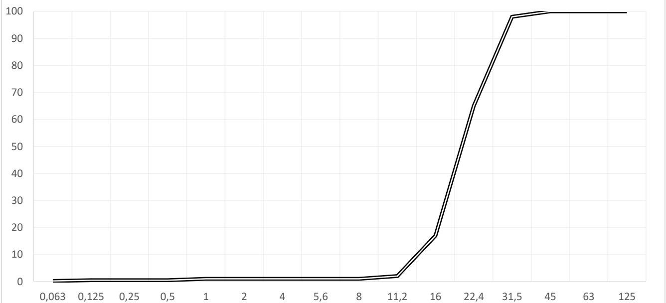
KORNSTORLEKSFÖRDELNING SS-EN 933-1
